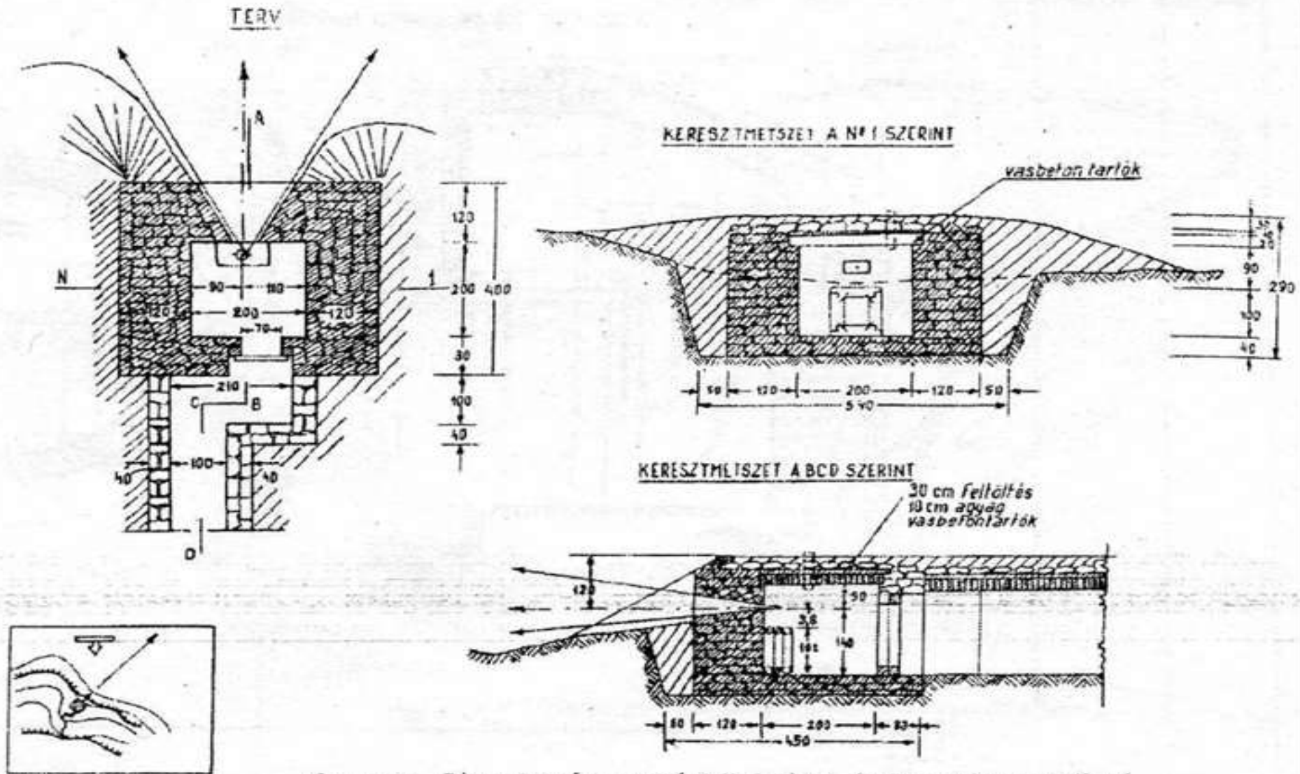
9.sz.rajz. Géppuskaerőd megerősített falakkal és könnyű típusu fodérmel.
